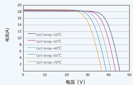
组件的I-V曲线 (665W)
