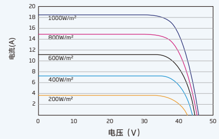
组件的P-V曲线 (665W)
